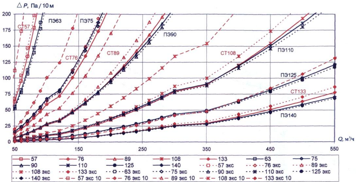
Удельные потери давления для стальных и полиэтиленовых труб (новых и бывших эксплуатации) низкого давления
